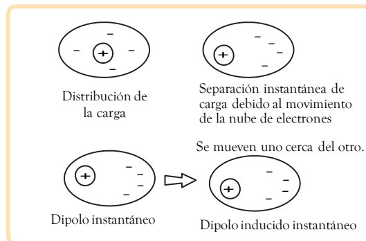
Fuerza de Dispersión de London
