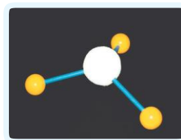
Molécula de \text{NH}_3
