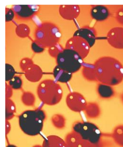
Fuerza de Dispersión de London
